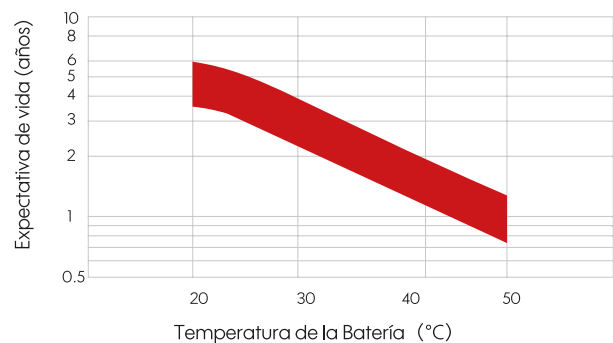
Efecto de la temp. en la vida útil de la batería en voltaje de flotación
