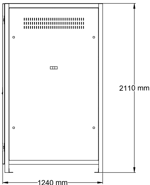
VISTA LATERAL
