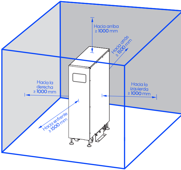
Figura 3-1 Requerimiento mínimo de espacio de instalación del AVR-IND 1300
