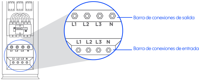
Figura 3-3 Barras de conexión del AVR-IND 1300
