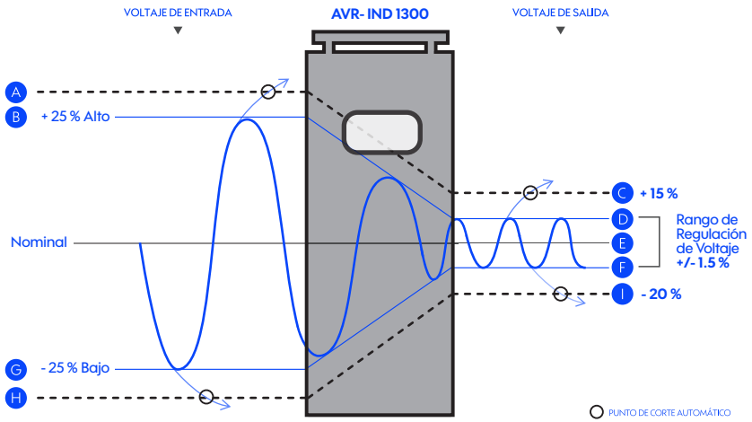
Figura 4-1 Embudo de regulación del AVR-IND 1300
