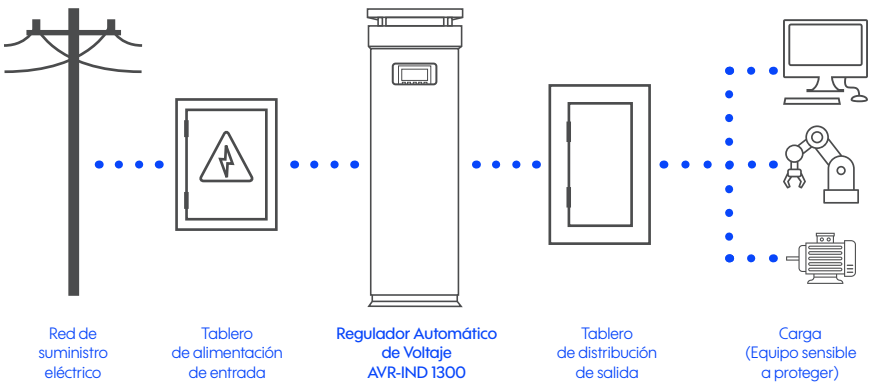
Figura 6-1 Diagrama de la instalación física del AVR-IND 1300
