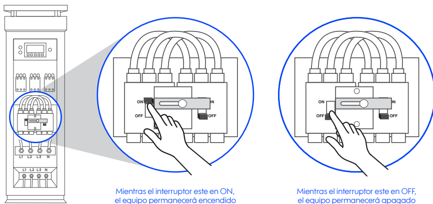
Figura 4-2 Ubicación del interruptor termomagnético de entrada para encender y apagar el AVR-IND 1300
