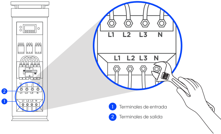
Figura 7-3 Conexiones de AVR-IND 1300
