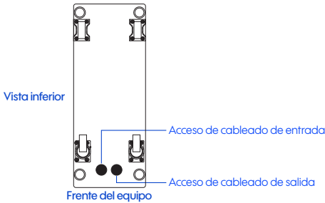
Figura 7-4 Acceso de cables de entrada y salida del AVR-IND 1300
