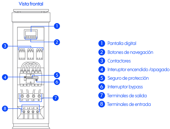
Figura 3-2 Componentes básicos AVR-IND 1300
