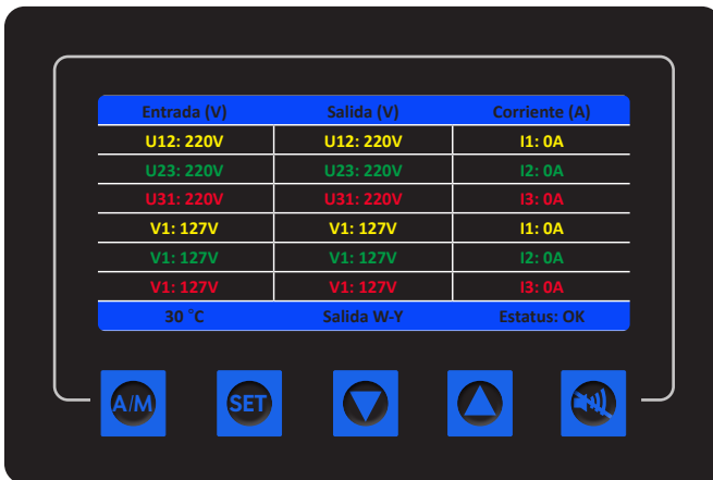
Figura 4-4 Pantalla LCD del AVR-IND 1300
