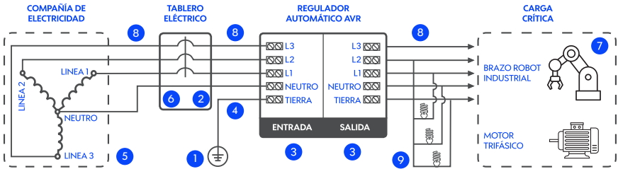
Figura 7-1 Sistema eléctrico trifásico para AVR-IND 1300
