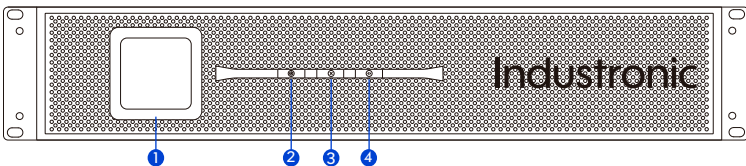
Figura 2-3 Tablero de control del UPS-IND 1100 RP
