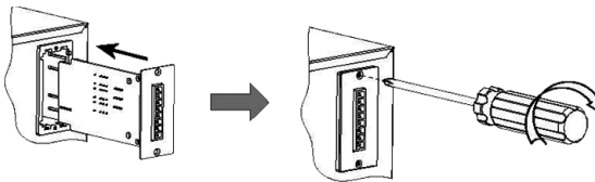
Figura 4-10 Instalación de la ranura inteligente opcional
