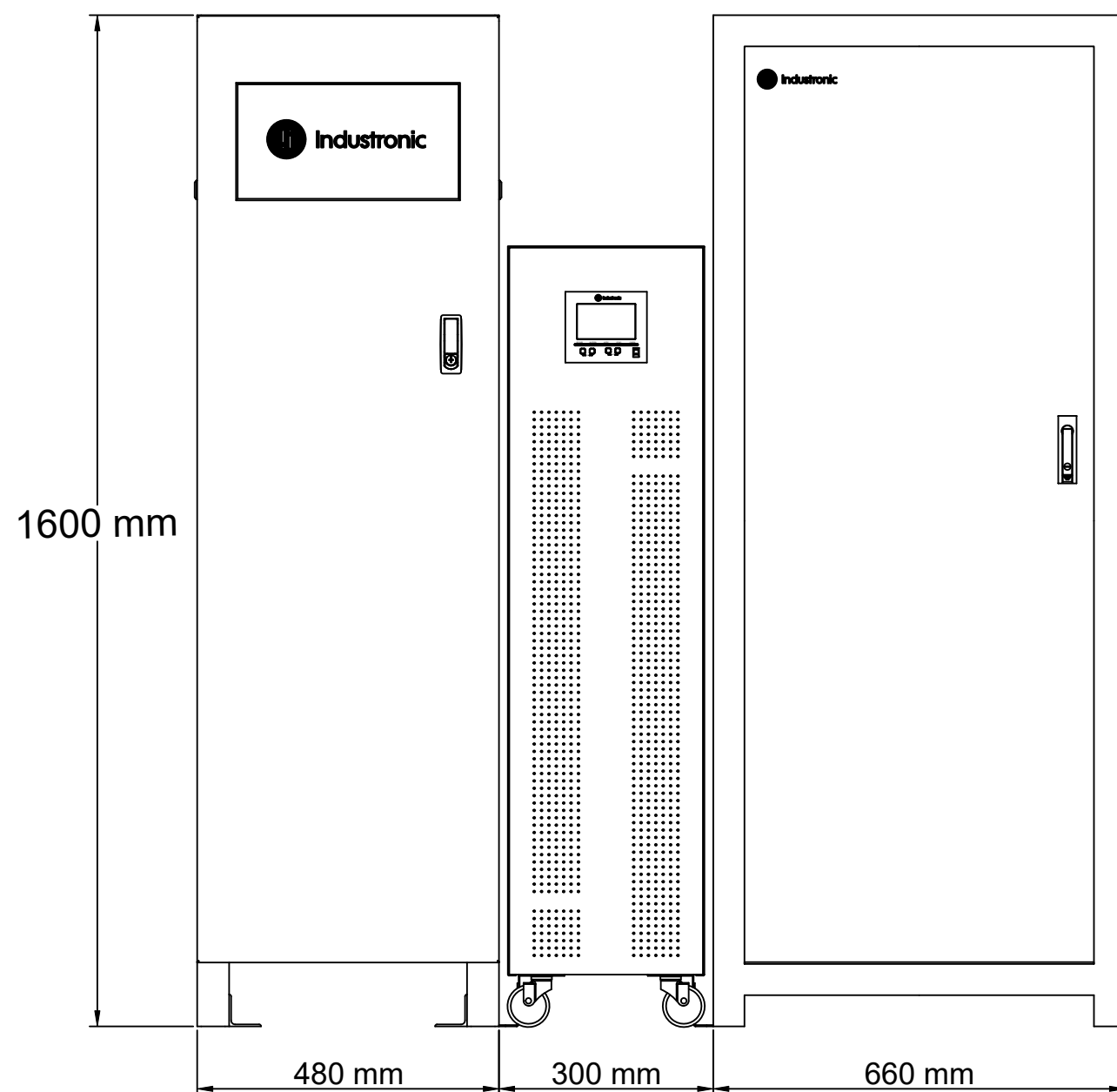
MOD. DE POT. UPS-IND HF 1340 M1 BAT-IND M1 1340
